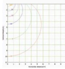
Dikey IsoLux Grafiği
